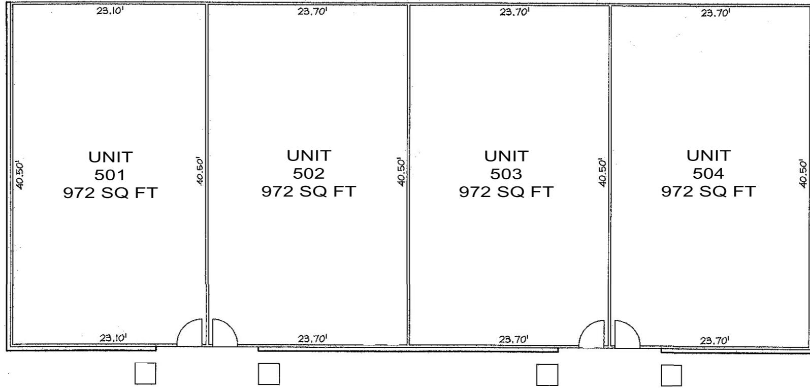
BLDG. V
